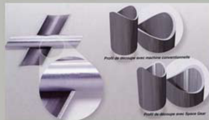
Découpe précise de tube rond selon un angle
